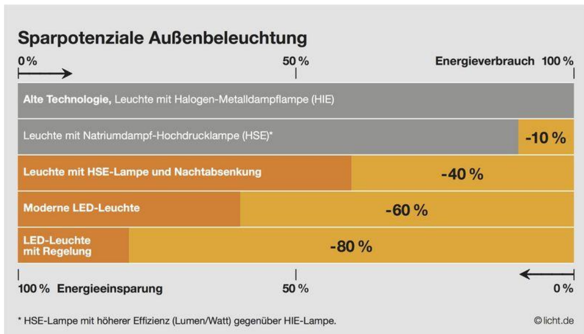
Abbildung 27: Energieeinsparpotenziale verschiedener Leuchtmittel im Außenbereich (Anonymus, 2019)
