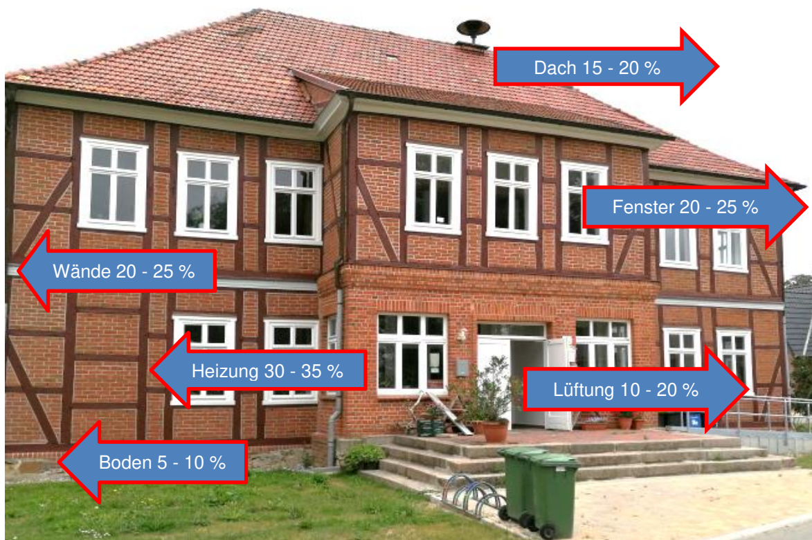
Abbildung 28: Mittlere Wärmeverluste eines Gebäudes mit einem Baujahr um 1980 (Baulink, 2010)
